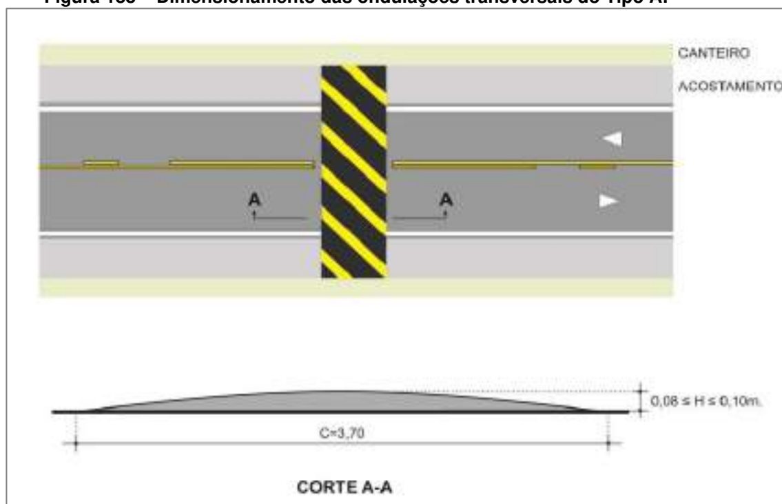
Figura 188 – Dimensionamento das ondulações transversais do Tipo A.
