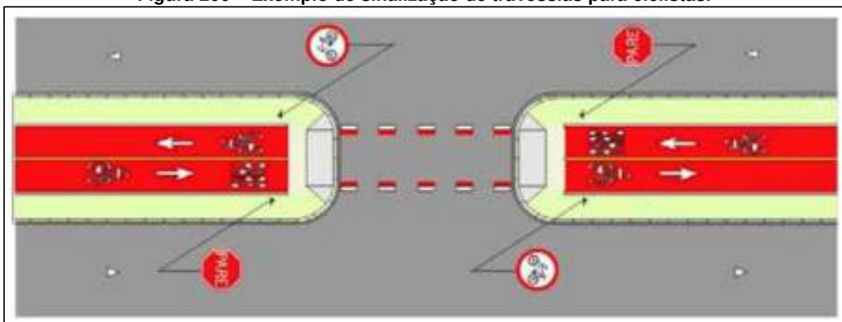
Figura 206 – Exemplo de sinalização de travessias para ciclistas.
