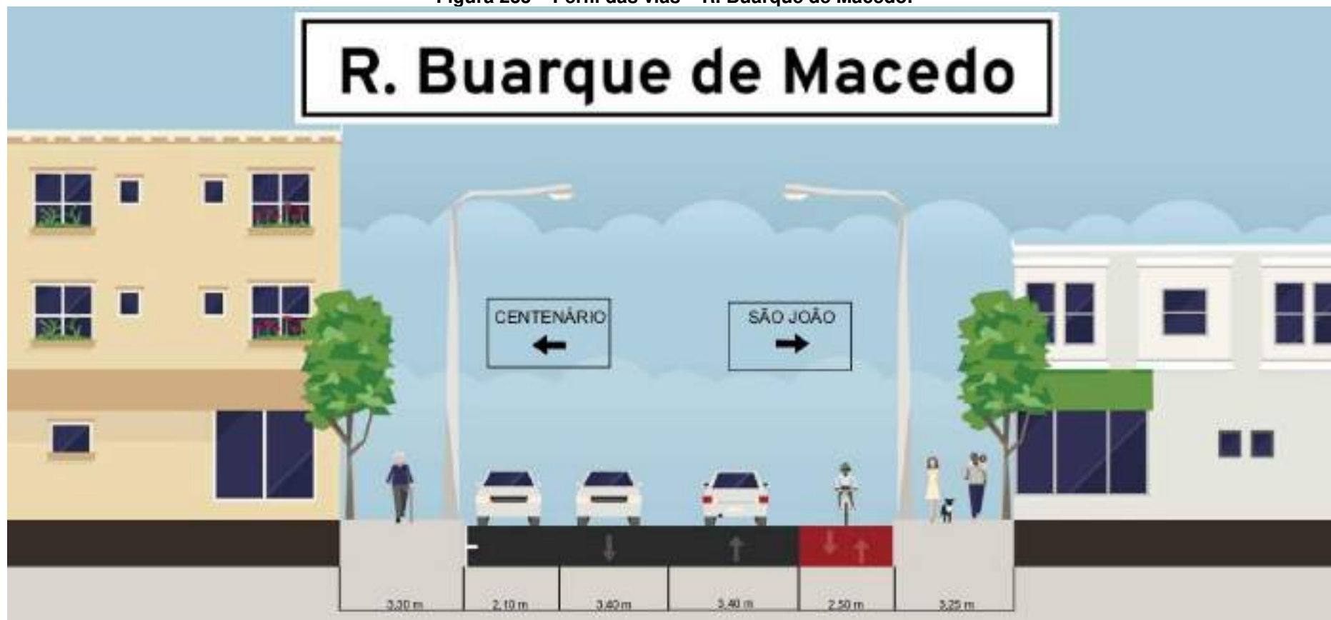
Figura 233 – Perfil das vias – R. Buarque de Macedo.
