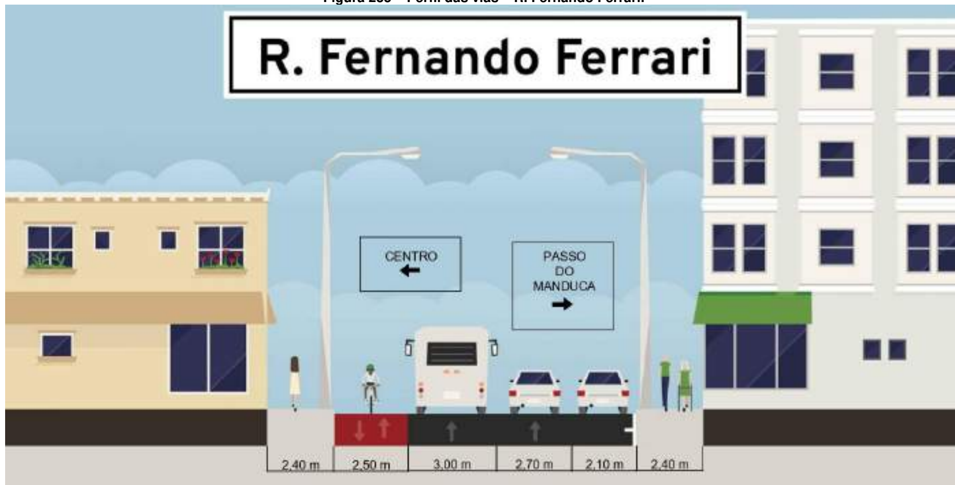
Figura 235 – Perfil das vias – R. Fernando Ferrari.
