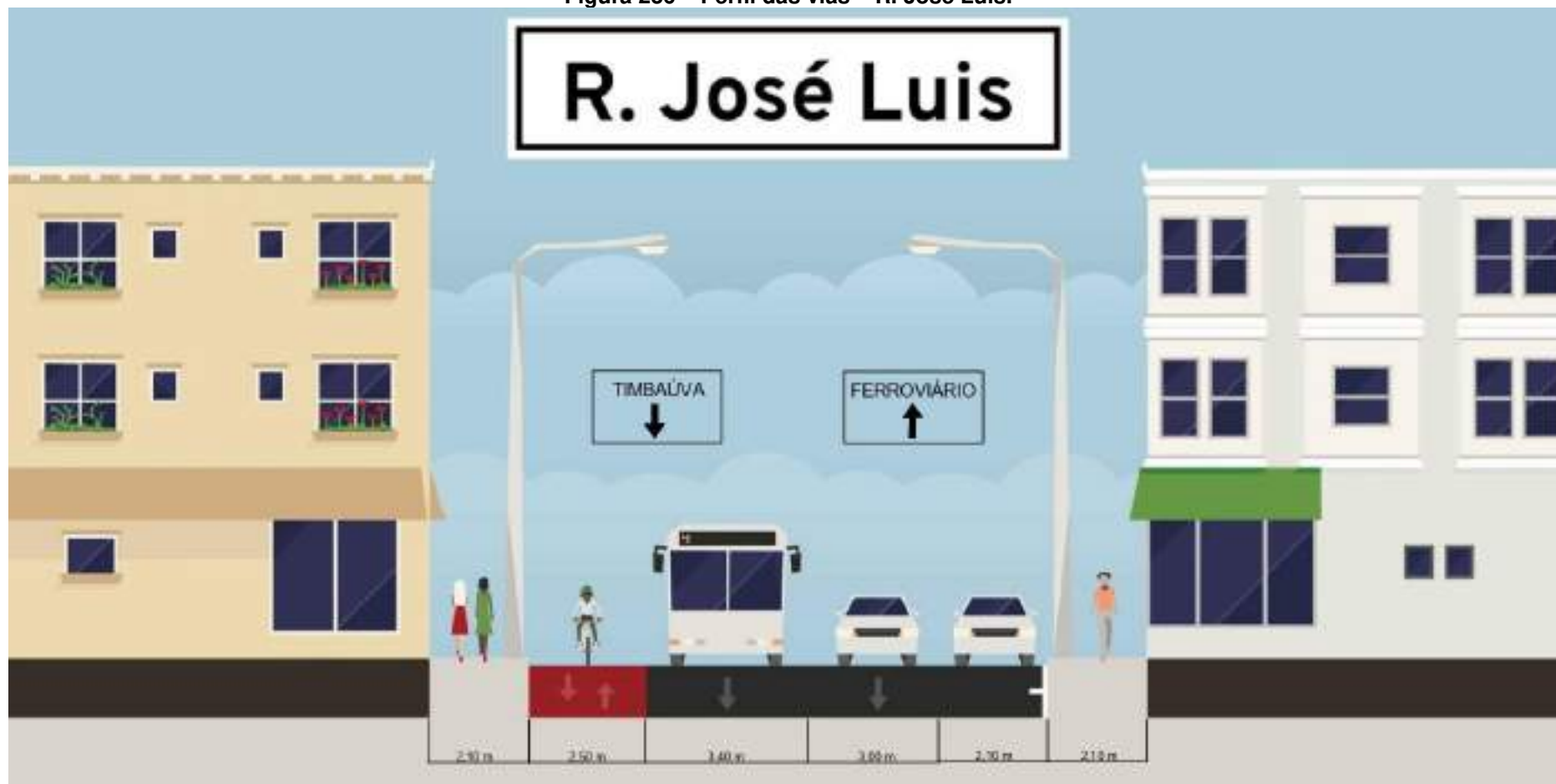
Figura 236 – Perfil das vias – R. José Luís.
