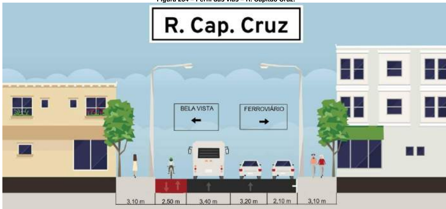
Figura 234 – Perfil das vias – R. Capitão Cruz.
