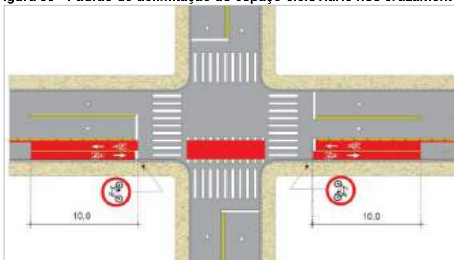
Figura 88 - Padrão de delimitação do espaço cicloviário nos cruzamentos
