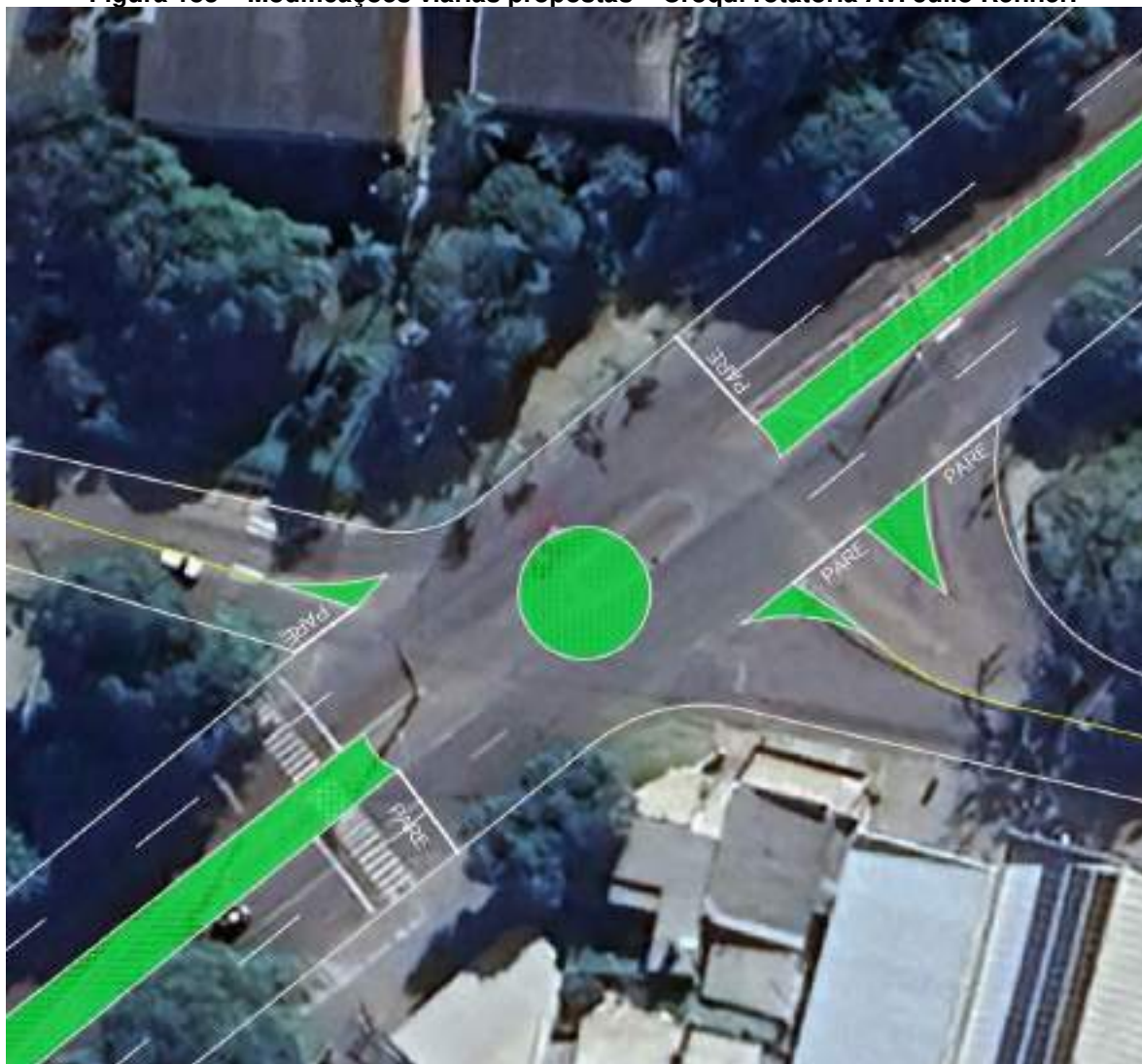
Figura 183 – Modificações viárias propostas – Croqui rotatória Av. Júlio Renner.
