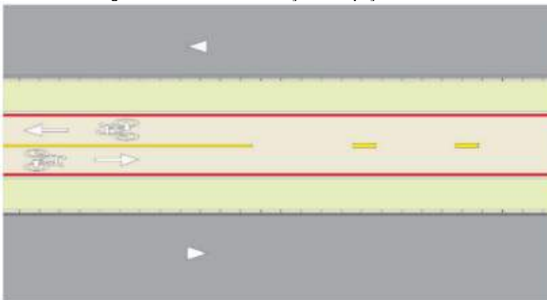
Figura 84 - Padrão de delimitação do espaço cicloviário
