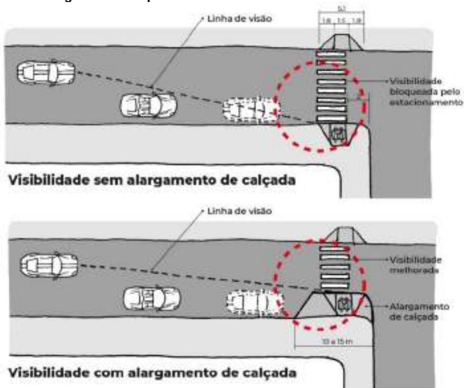
Figura 74 – Esquema de visibilidade em cruzamentos.
