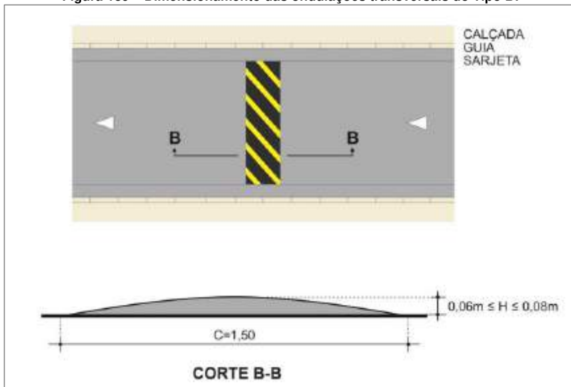
Figura 189 – Dimensionamento das ondulações transversais do Tipo B.
