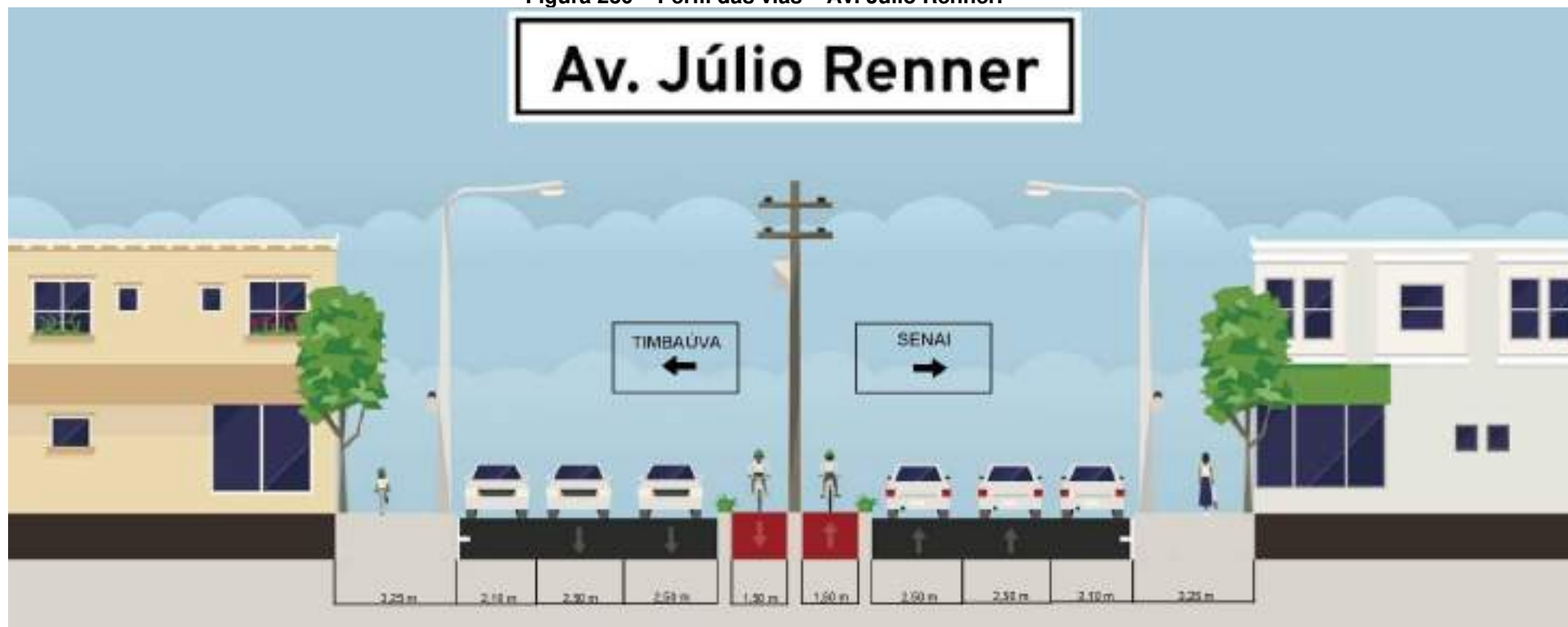
Figura 230 – Perfil das vias – Av. Júlio Renner.
